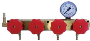
circuit mesure
